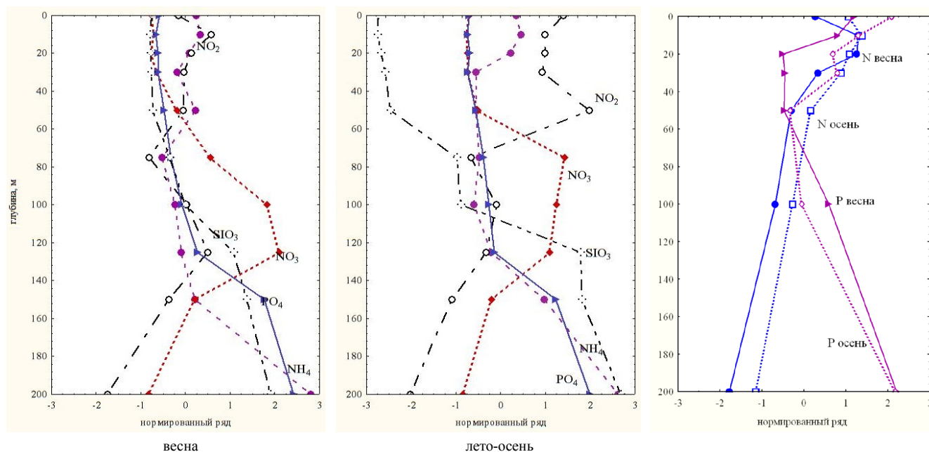
Рис. 2. Вертикальная структура экстремумов биогенных веществ в северо-восточной части Черного моря по многолетним данным 1996–2018 гг. по сезонам
